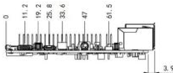
侧视图
